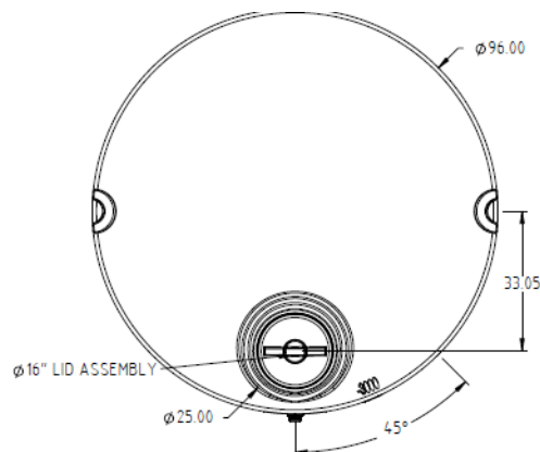
LID FOR VT2500-96 & VT3000-96
