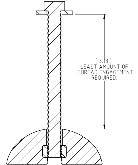
SECTION A-A SCALE 1:15
