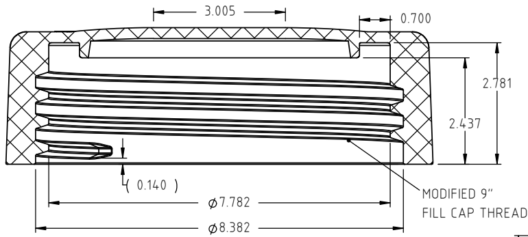
SECTION A-A SCALE 1:3
