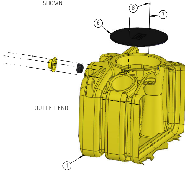
OPTIONAL BURIAL LID ASSEMBLY P.N.= ACT-16053BK SHOWN
