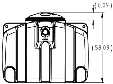
OPTIONAL BURIAL LID ASSEMBLY P.N.= ACT-16053BK SHOWN
