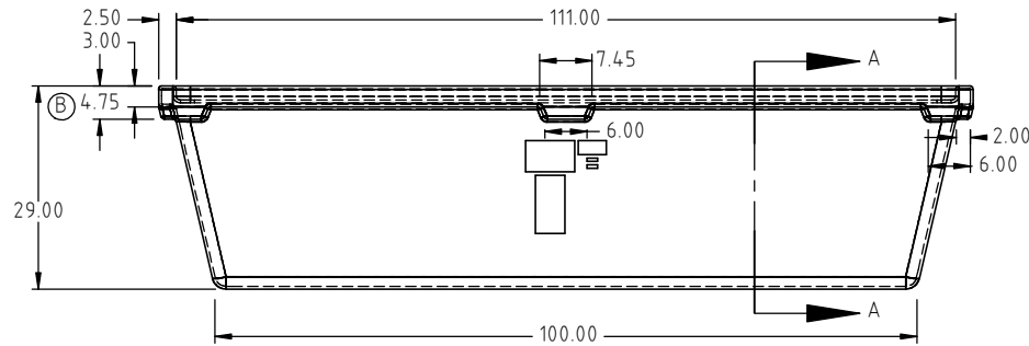
SECTION A-A SCALE 1:30
